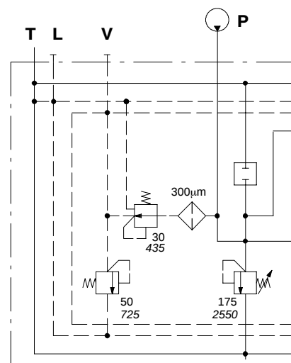
Description example: CRV(TVG3-175)....- TAP(VL)-SAE
