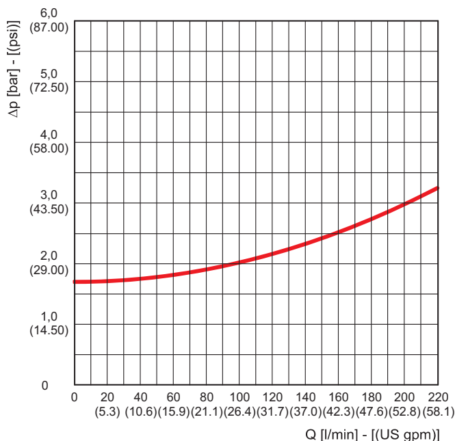
HF 650-30 (B17)
