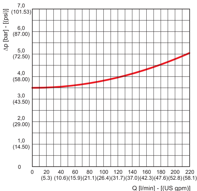
HF 650-30 (B35)
