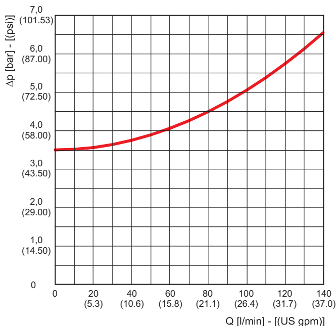
HF 650-20 (B35)
